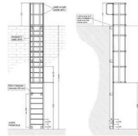
PARTICOLARE SCALA ALLA MARINARA
